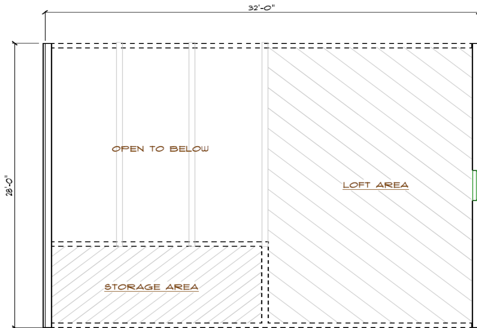
The Kennebago 2 Loft Plan 232 Sq. Ft.
